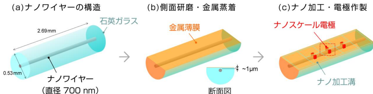
図 1 石英ガラス中のビスマスナノワイヤー上への電極作製プロセス
